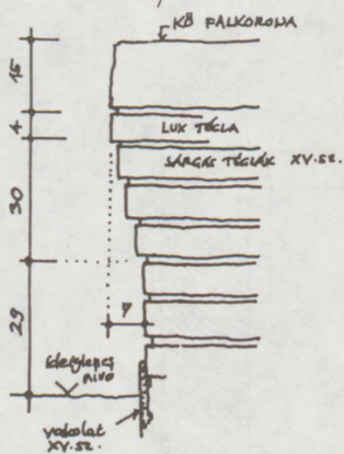
② METSZET
