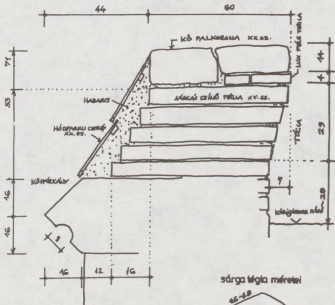
② METSZET
